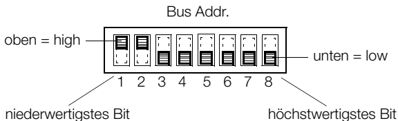
Bild 14 Beispiel Bus-Adresse = 3
