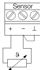
Pt100 2-Leiter
