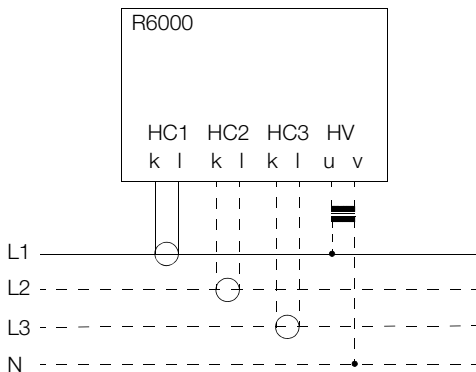
Bild 9 Prinzipschaltbild Stromwandleranschluss
