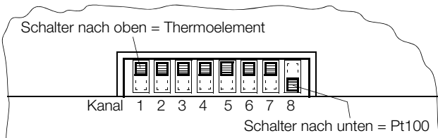
Bild 3 Fühlertyp-Einstellung
