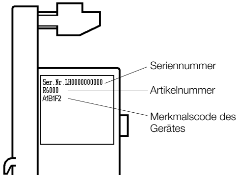
Bild 1 Typschildbeschriftung
