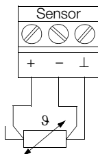
Pt100 3- bzw. 4-Leiter
