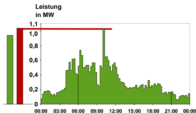
Bezugsprofil
