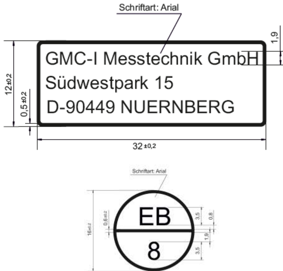
Abb. 2 Siegetikett für Zugriffssicherung (Angaben in mm)
