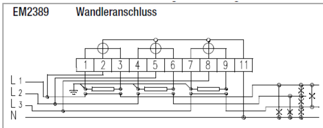
Abb. 7 Anschlussschaltbilder
